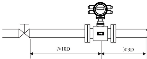
图 10 阀门位于传感器上游的安装
