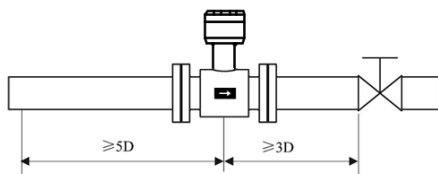
图7 阀门位于传感器下游的安装
