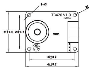
俯视图
