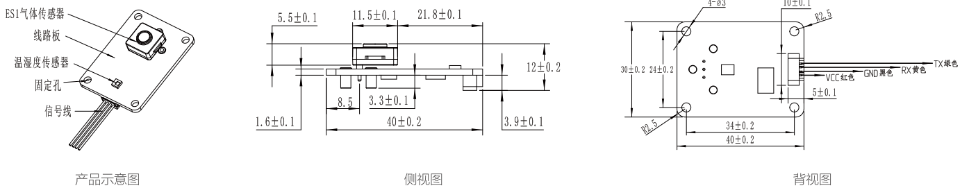
TB200B-ES1-CO-10-01尺寸示意图
