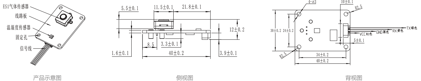
TB200B-ES1-CO-100-01尺寸示意图
