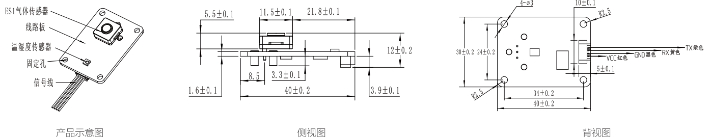
TB200B-ES1-CO-2%-01尺寸示意图
