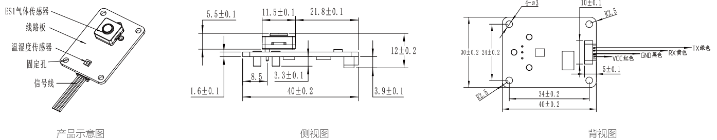
TB200B-ES1-O 2 -25%-01尺寸示意图
