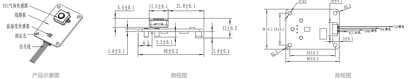
TB200B-ES1-H 2 -1000-01尺寸示意图
