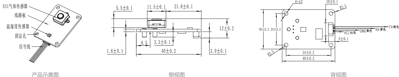
TB200B-ES1-H 2 S-100-01尺寸示意图
