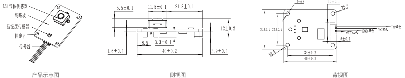
TB200B-ES1-NO 2 -100-01尺寸示意图
