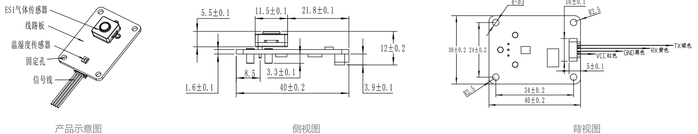
TB200B-ES1-NO 2 -5-01尺寸示意图
