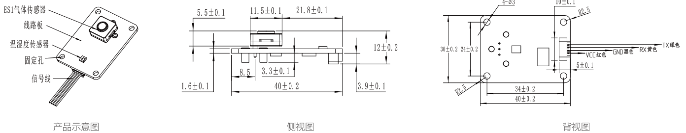
TB200B-ES1-NO 2 -50-01尺寸示意图
