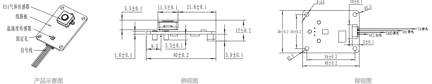
TB200B-ES1-O 3 -5-01尺寸示意图
