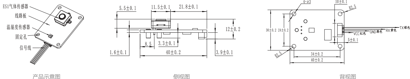
TB200B-ES1-O 3 -100-01尺寸示意图
