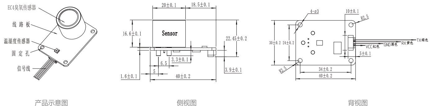
TB200B-EC4-O 3 -100-01尺寸示意图
