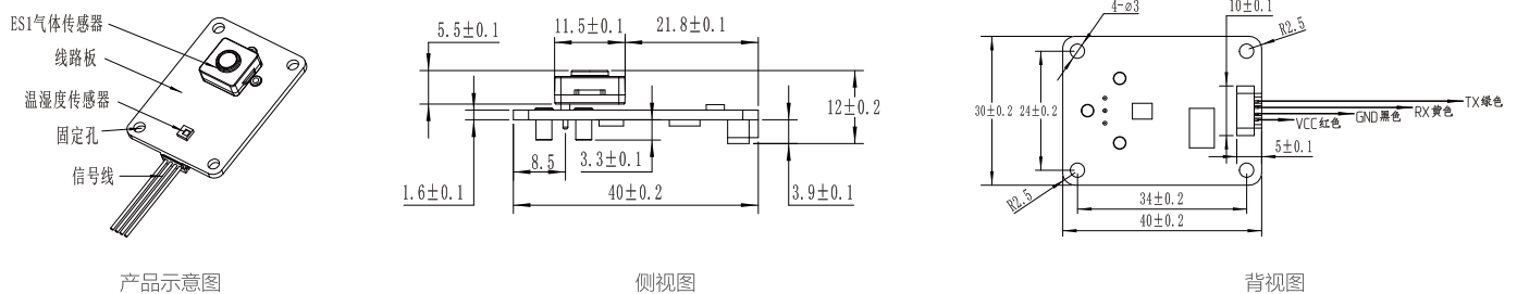
TB200B-ES1-SO 2 -100-01尺寸示意图
