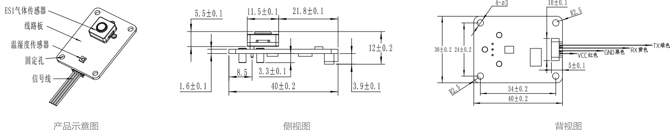
TB200B-ES1-SO 2 -1000-01尺寸示意图
