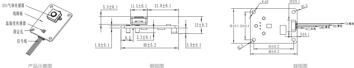
TB200B-ES1-SO 2 -5-01尺寸示意图
