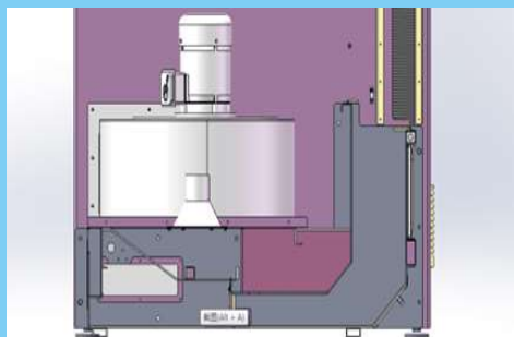
L型吸风箱
