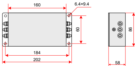
图 7-3 竖力滤波器 DL-10EBK5/ DL-16EBK5 尺寸图 (单位: mm)
