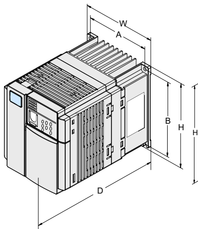
0.4kW-2.2kW 外形及安装尺寸示意图
