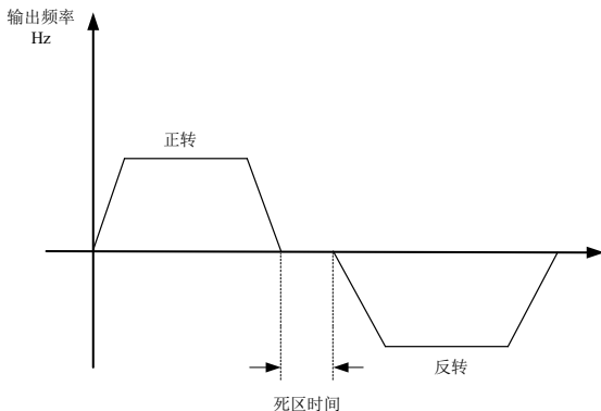
图 6-21 正反转死区时间示意图
