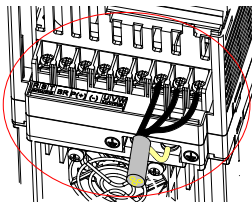
图 7-6 屏蔽电缆接地示意图
