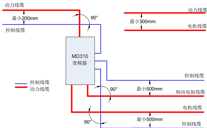
图 7-7 电缆布线图
