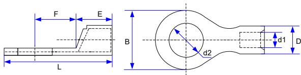
图 3-11 TNR 系列圆型线耳外观及尺寸图（推荐）
