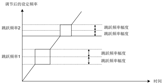
图 6-20 跳跃频率示意图
