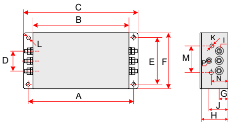
图 7-3 竖力滤波器 DL-25EBK5/ DL-35EBK5/ DL-50EBK5 尺寸图
