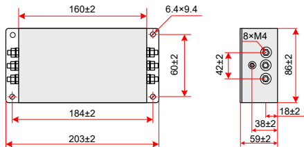
图 7-2 竖力滤波器 DL-5EBK5 尺寸图 (单位: mm)
