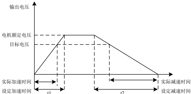
图 6-6 V/F 分离示意图
