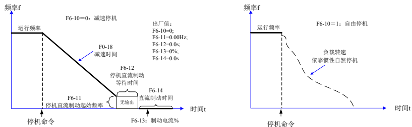
图 4-12 停机模式
