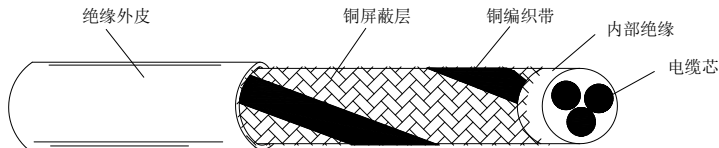
图 7-5 屏蔽层的编织密度
