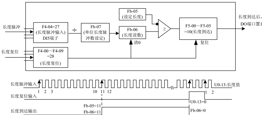
图 4-24 定长控制模式功能码设置
