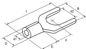
图 3-12 TNS 系列叉形线耳外观及尺寸图（【注】）
