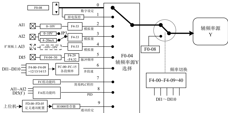
图 4-18 辅助频率给定来源选择
