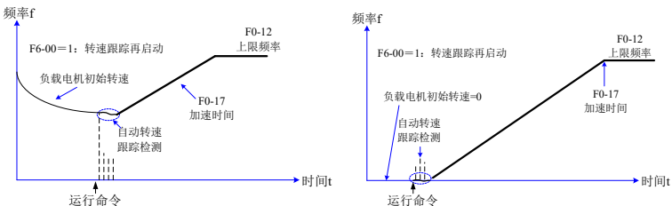
图 4-10 速度跟踪再启动方式
