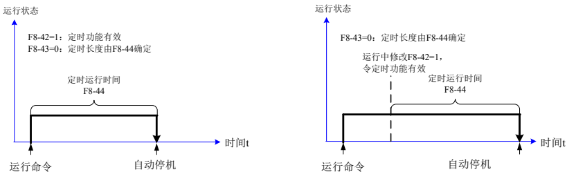
图 4-13 定时停机功能
