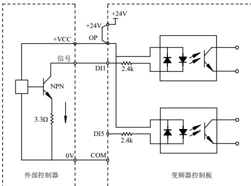
图 3-16 漏型接线方式
