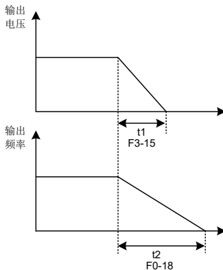
图 6-7 V/F 分离输出电压 / 频率独立减至 0
