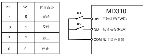
图 6-12 两线式模式 1
