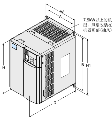
3.7kW-18.5kW 外形及安装尺寸示意图
