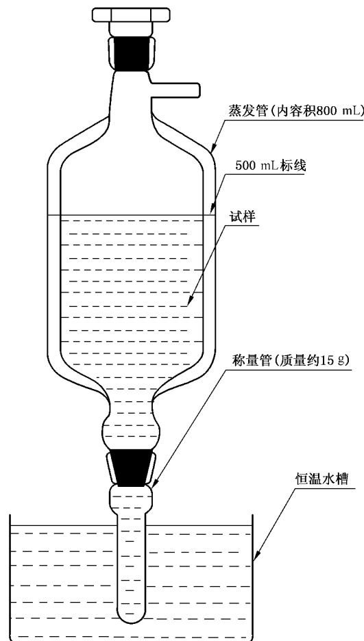
图 1 蒸发器
