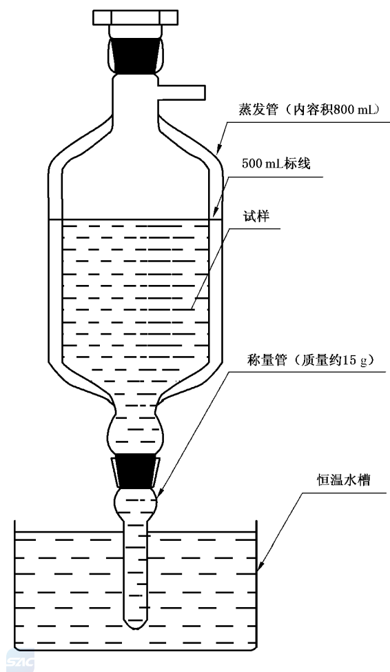
图 1 蒸发器
