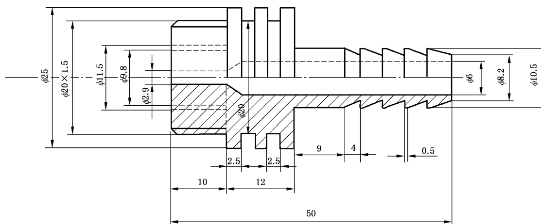
b) 喷嘴芯
