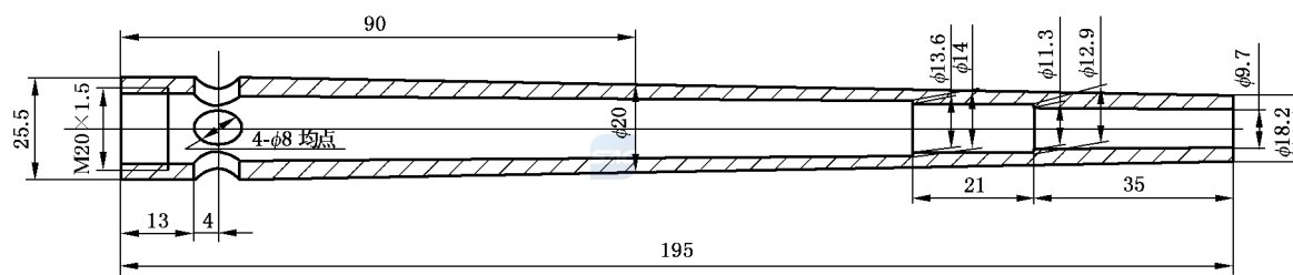
a) 喷嘴
