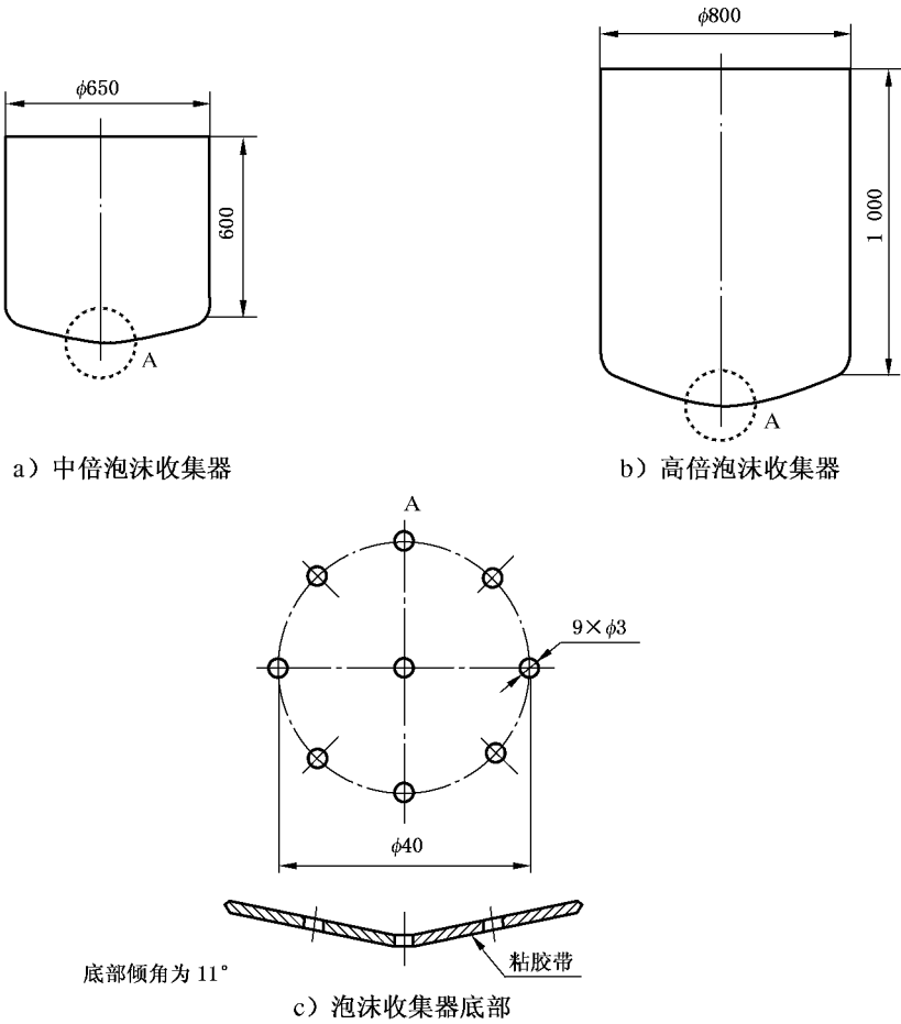
图 6 泡沫收集器
