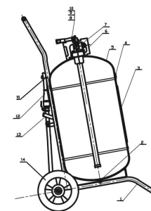
结构示意图 STRUCTURE DIAGRAM
