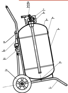
结构示意图 STRUCTURE DIAGRAM
